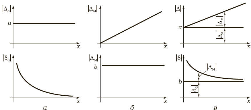
Рис. 7.2. Абсолютные погрешности: a — аддитивная; б — мультипликативная; в — суммарная
