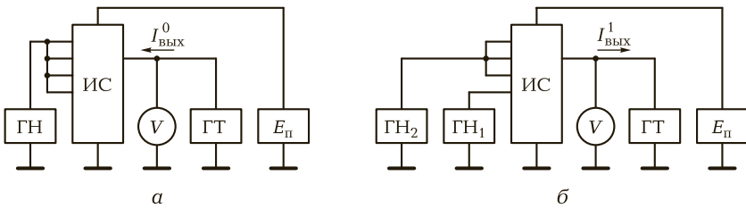
Рис. 10.9. Схемы для измерения выходного напряжения логического нуля и логической единицы:
