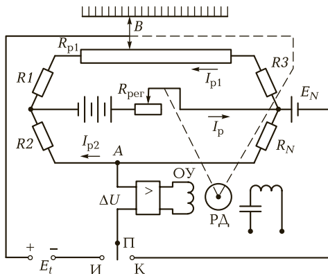
Рис. 11.5. Схема автоматического потенциометра постоянного тока
