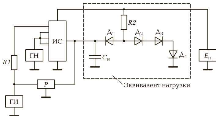
Рис. 10.13. Схема измерения динамических параметров
