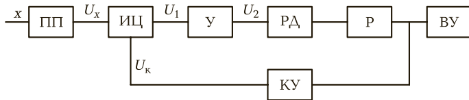
Рис. 11.3. Структурная схема АИП непрерывного действия
